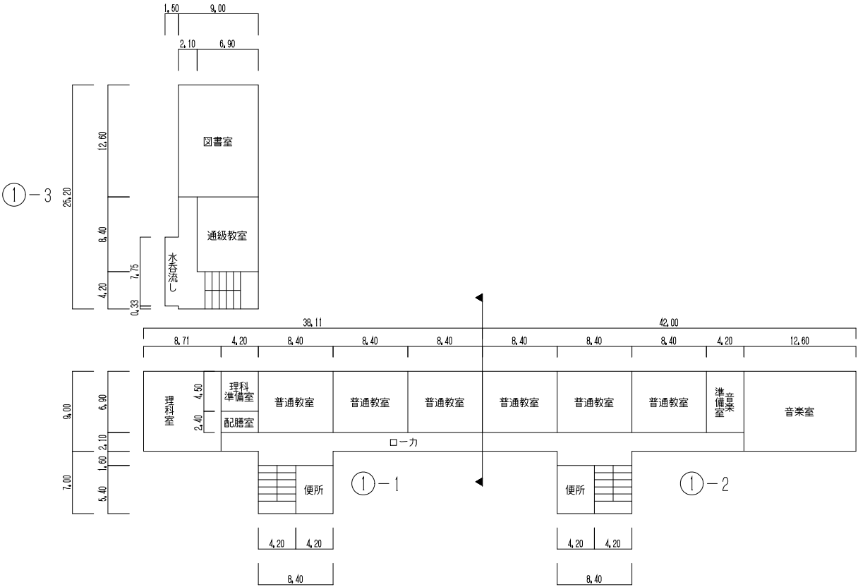
2 階 平 面 図
