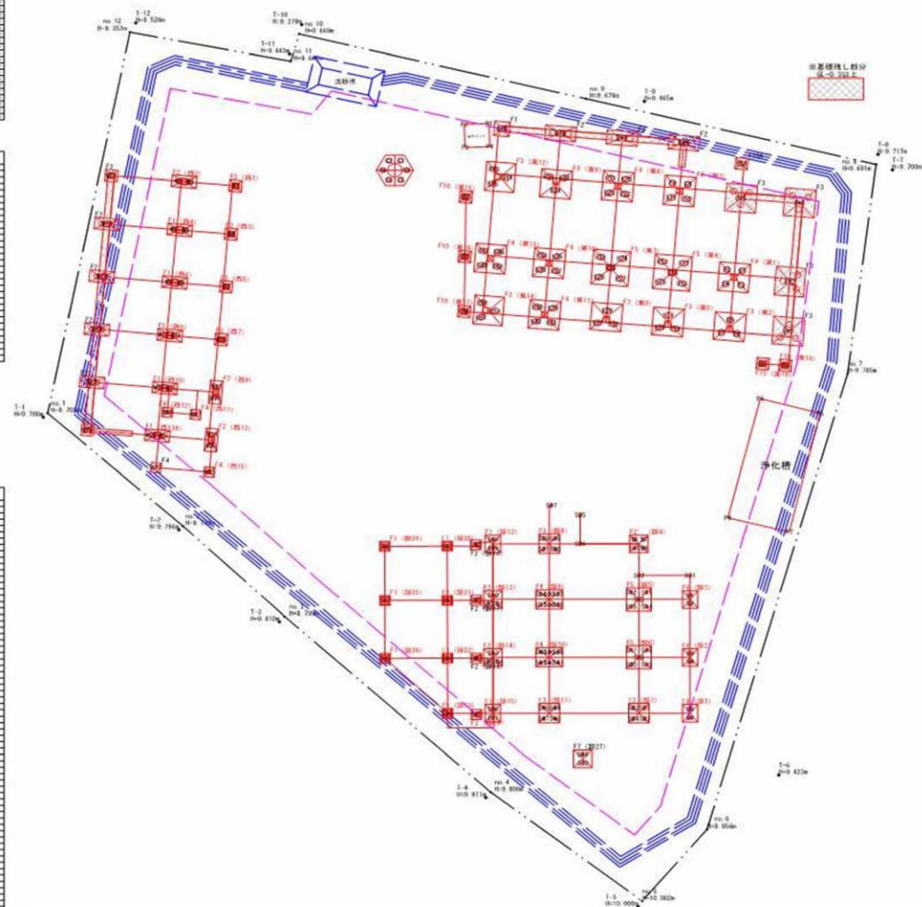
13 地下埋設物 平面図
